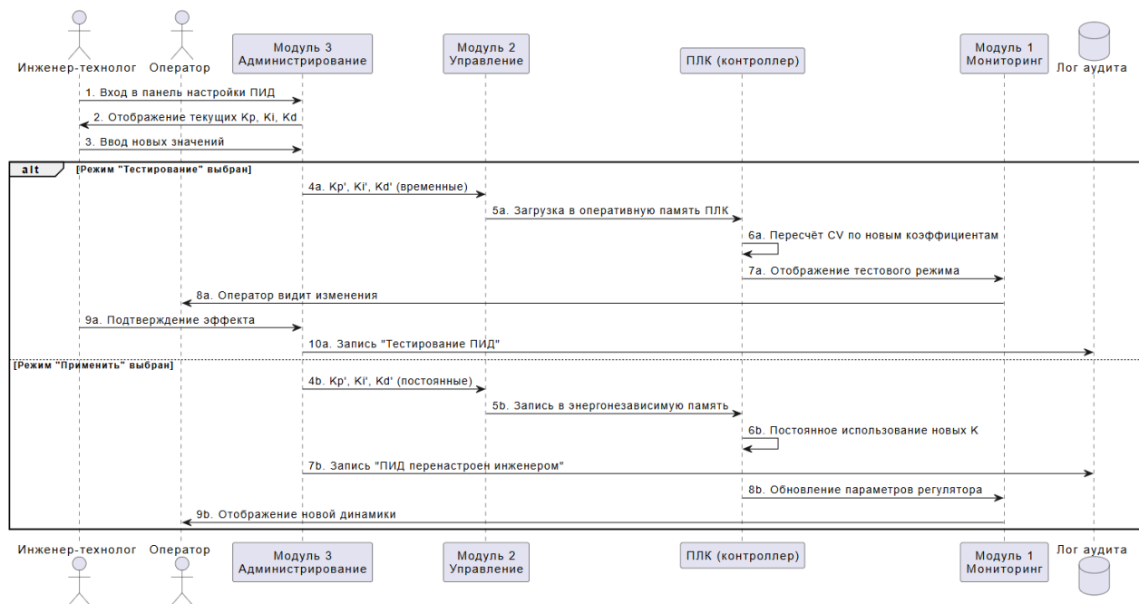
Рисунок 3 - Процесс 3: Настройка ПИД-коэффициентов инженером-технологом
