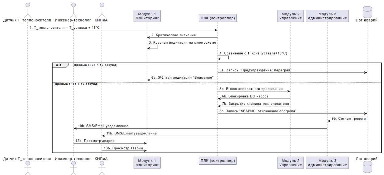
Рисунок 2 - Процесс 2: Защитное отключение подпочвенного обогрева при перегреве
