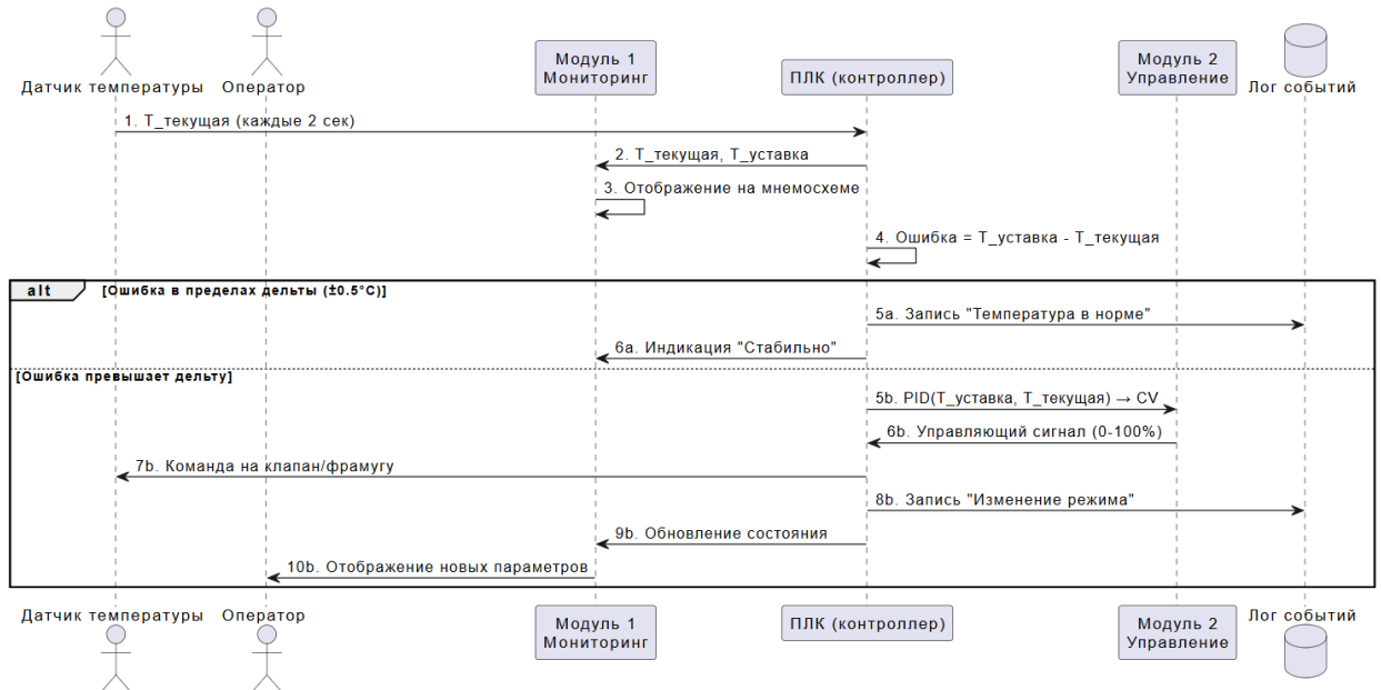
Рисунок 1 - Процесс 1: Автоматическое ПИД-регулирование температуры в климатической зоне
