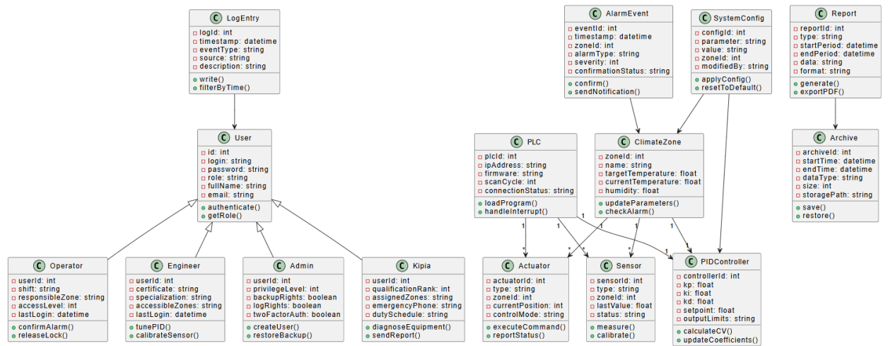
Рисунок 4 - Диаграмма классов
